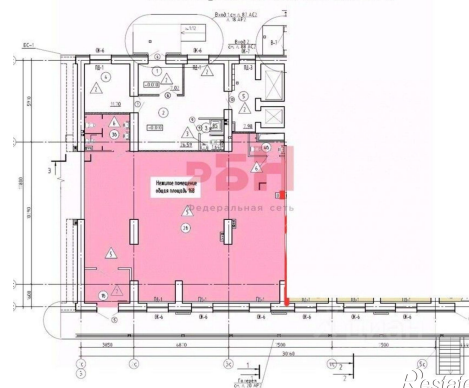
План первого этажа, секция БС-2
